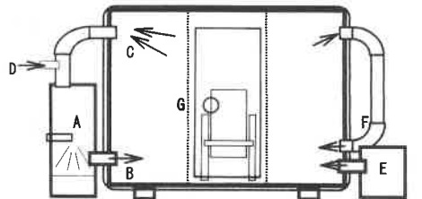
A: 真気発生装置、B: 真気ダクト、C: 真気用換気口、D: 外気吸入口、E: 湿式サウナ装置、F: 湿式サウナ用換気ダクト、G: 被験者出入用扉 真気サウナの構造
